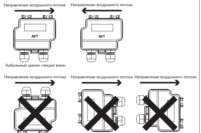
Рисунок 1с - Направление монтажа
