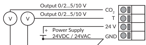
Рисунок 2с - Монтажная электросхема: дополнительный заземленный кабель
