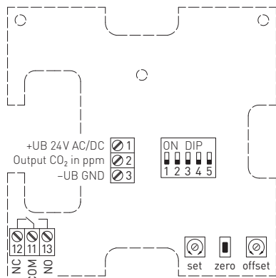
Схема подключения
