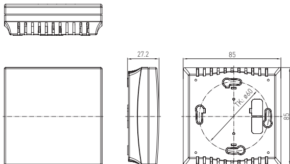
Габаритный чертеж
