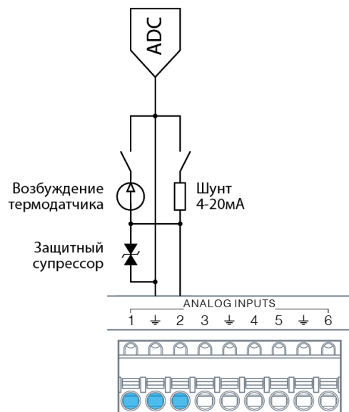
Рис. 19 – Внутренняя структура аналоговых входов
