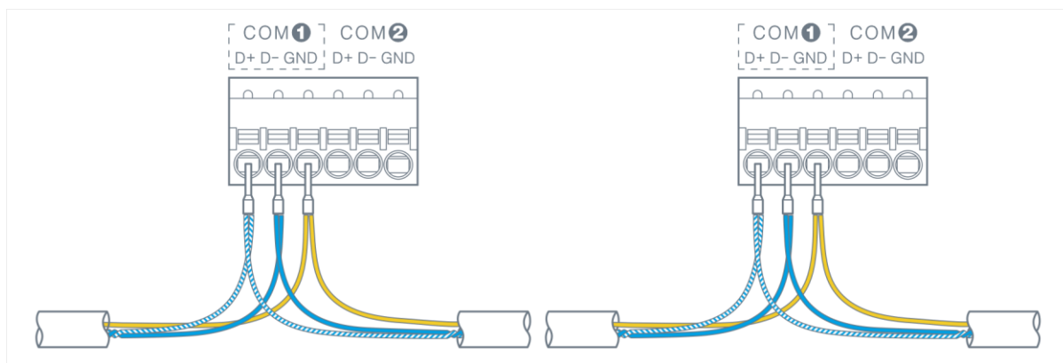
Рис. 28 - Организация подключения проводников RS-485
