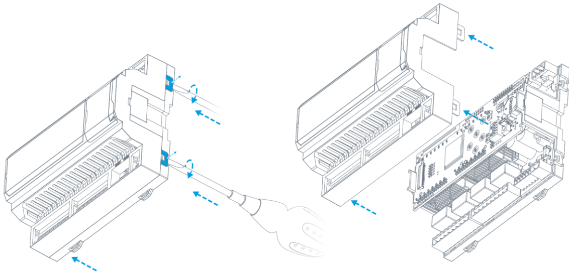
Рис. 47 – Открытие корпуса
