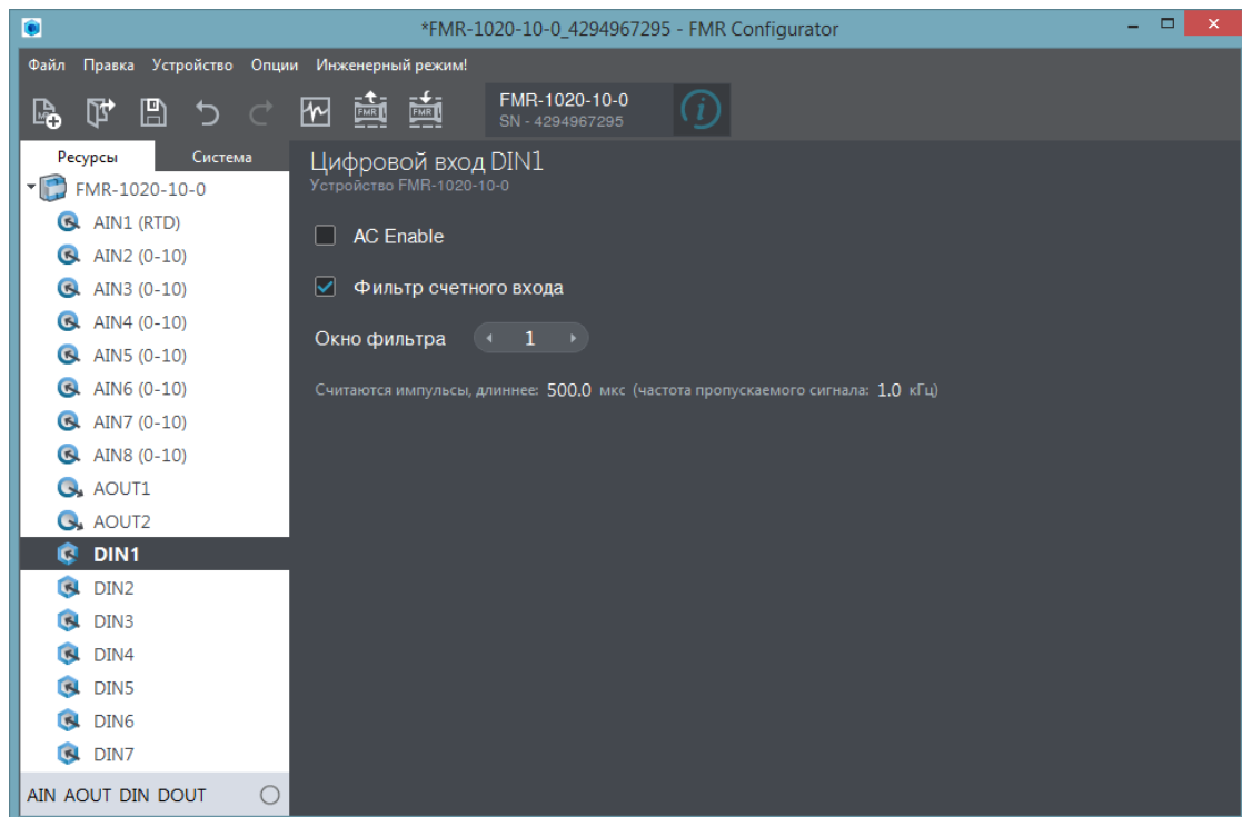
Рис. 39 – Конфигурация DIN
