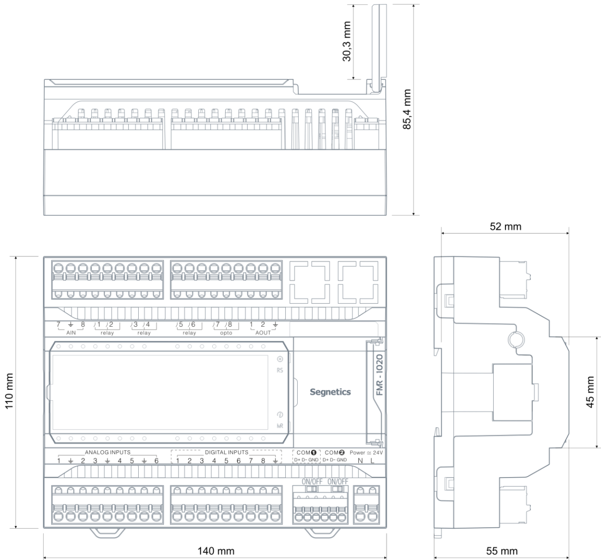
Рис. 4 - Габаритные и установочные размеры модуля
