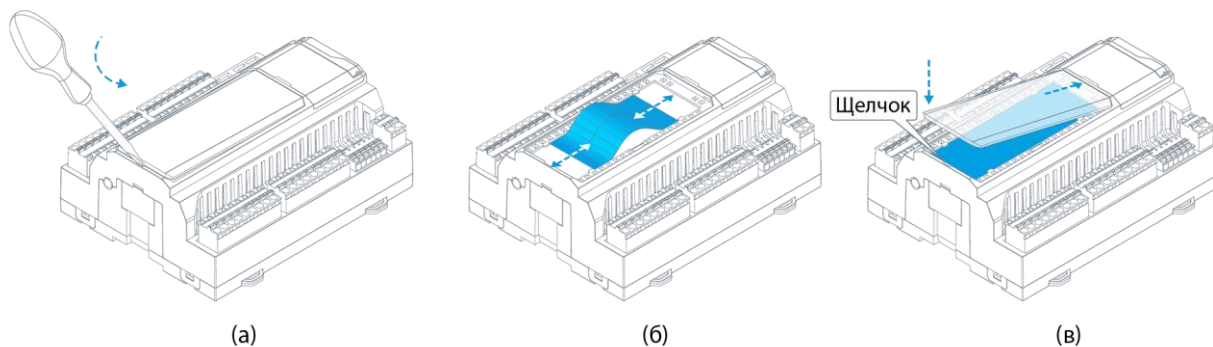
Рис. 9 – Извлечение и установка маркировочного шаблона.
