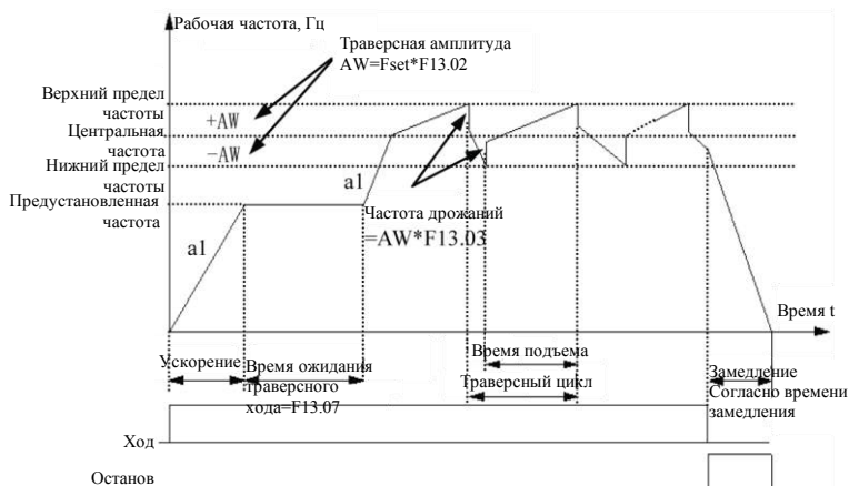
Рис.7-43 Траверсный ход
