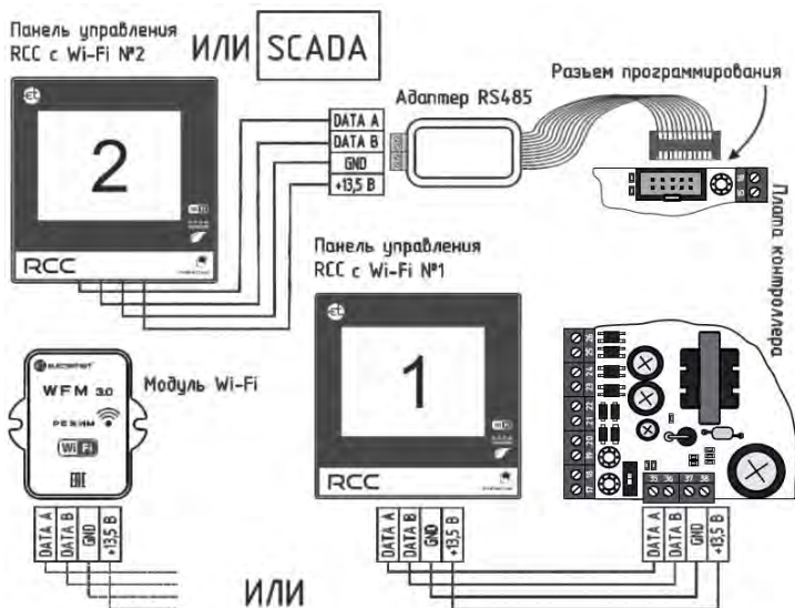
Рис.2.2 Подключение средств ДУ
