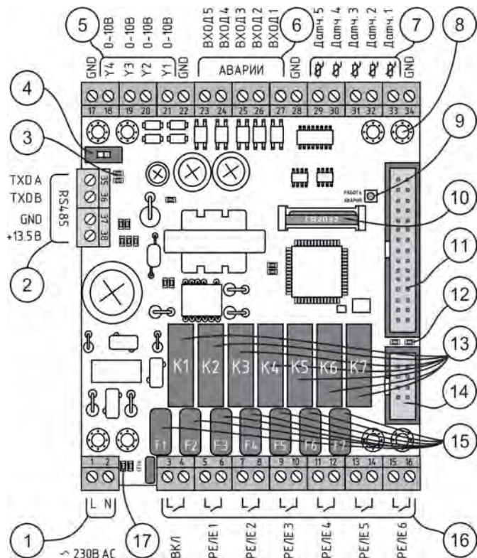
Рис. 1.1. Основные элементы и элементы индикации контроллера
