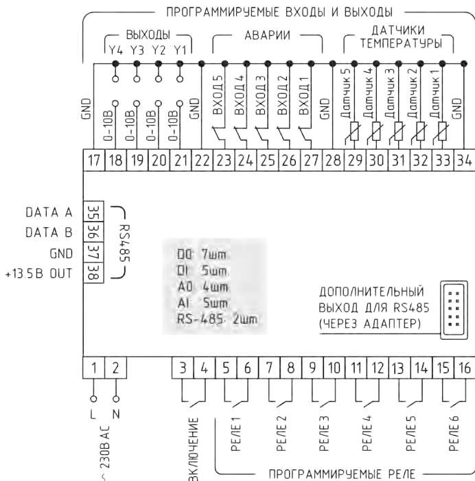
Рис. 2.1 Назначение клемм контроллера.
