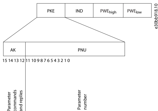
Рисунок 47: Поле PKE
