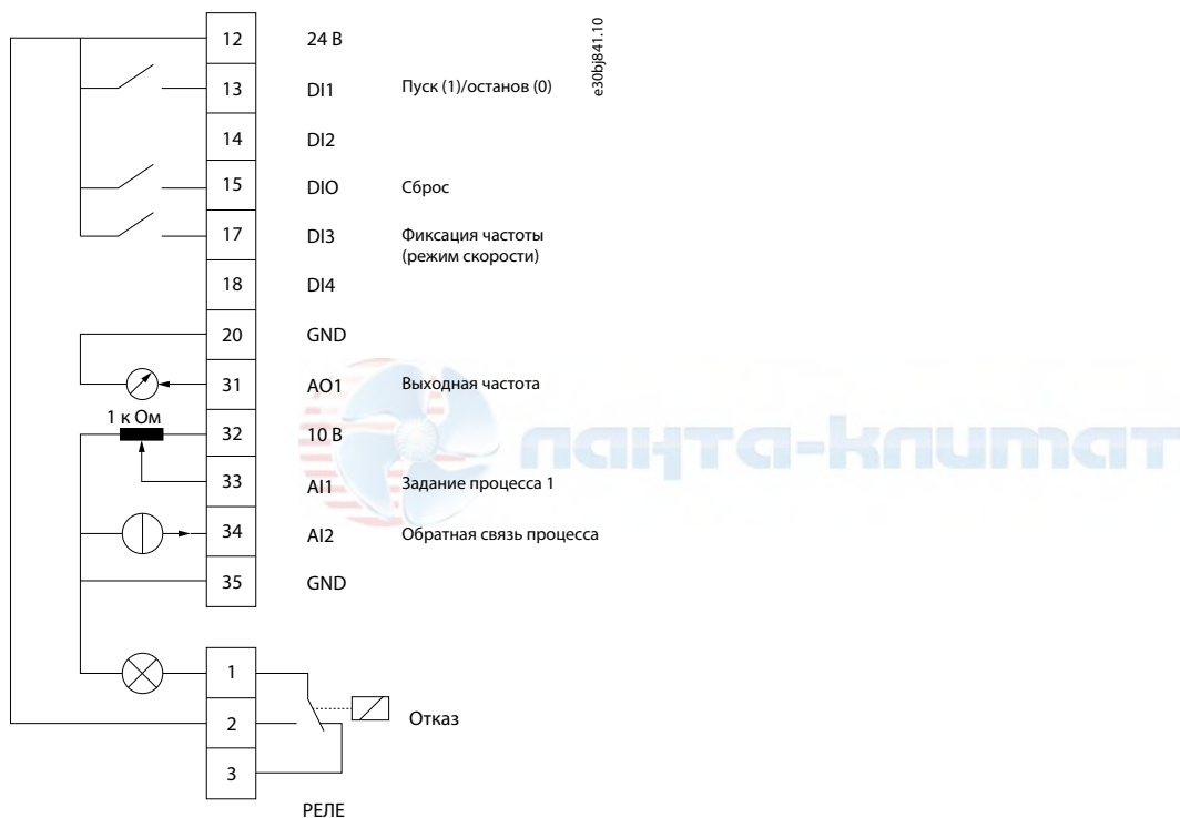
Рисунок 25: Подключения по умолчанию для управления процессом
