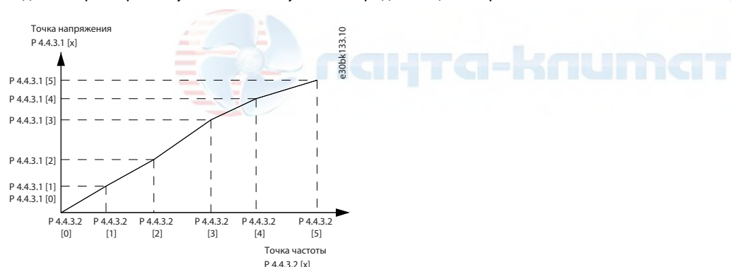
Рисунок 57: Пример характеристики U/f
