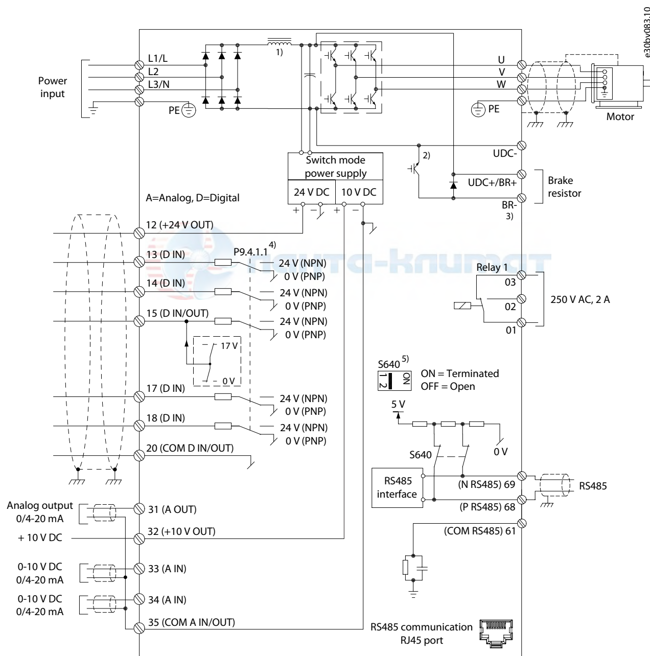
Рисунок 22: Схема соединений
