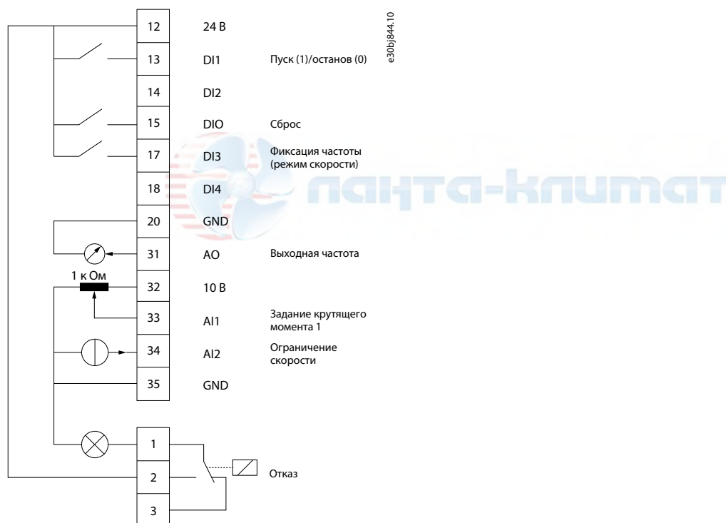
Рисунок 29: Цепи управления, используемые по умолчанию
