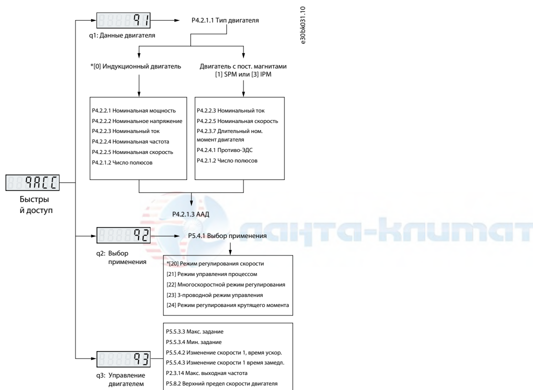
Рисунок 4: Функции быстрого доступа
