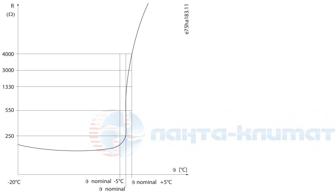
Рисунок 59: Профиль РТС
