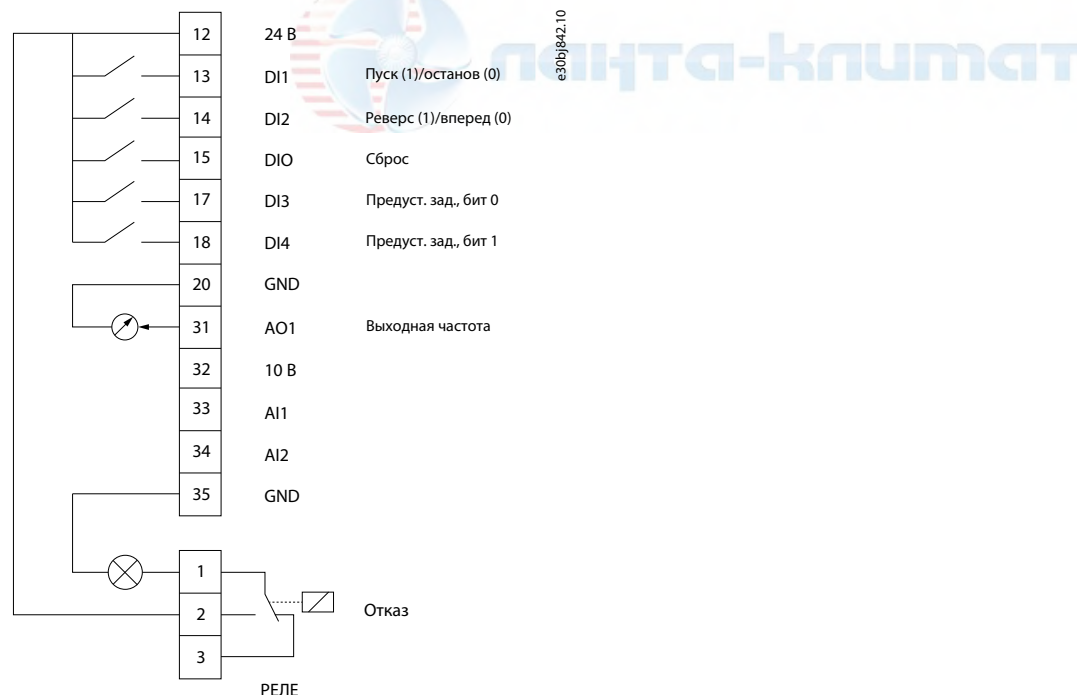
Рисунок 26: Цепи управления, используемые по умолчанию
