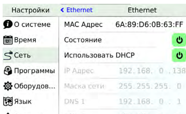
Рис. 26 – Редактор настроек интерфейса Ethernet.
