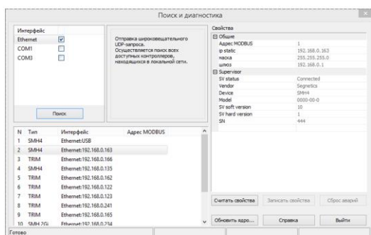
Рис. 95 – Окно «Поиск и диагностика со списком найденных контроллеров»
