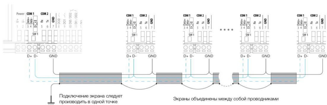
Рис. 43 – Экранирование сети RS-485
