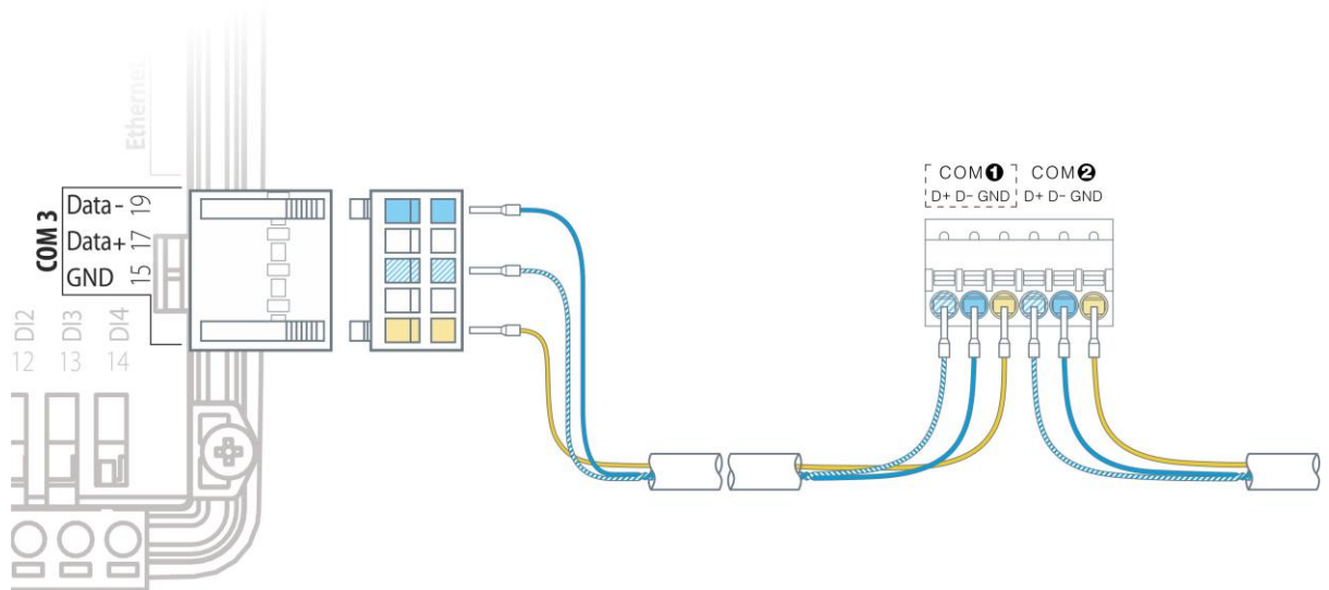
Рис. 52 –Порядок подключения проводов шины MTBus
