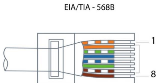
Рис. 53– Нумерация проводников в кабельном разъёме Настройка параметров порта
