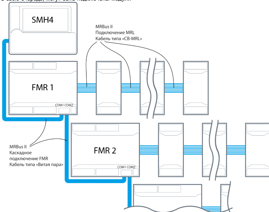
Рис. 51 – Организация шины MTBus
