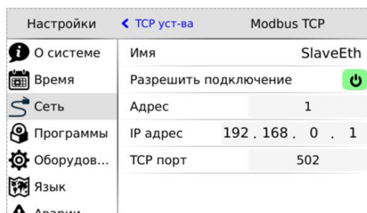
Рис. 71 – Настройка Modbus-TCP slave
